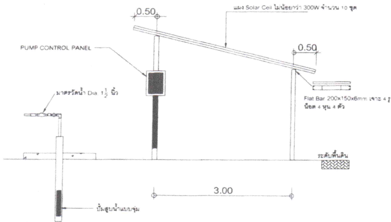
แบบร่างระบบสูบน้ำพลังงานแสงอาทิตย์ ขนาดรวมไม่น้อยกว่า 3,000 วัตต์
